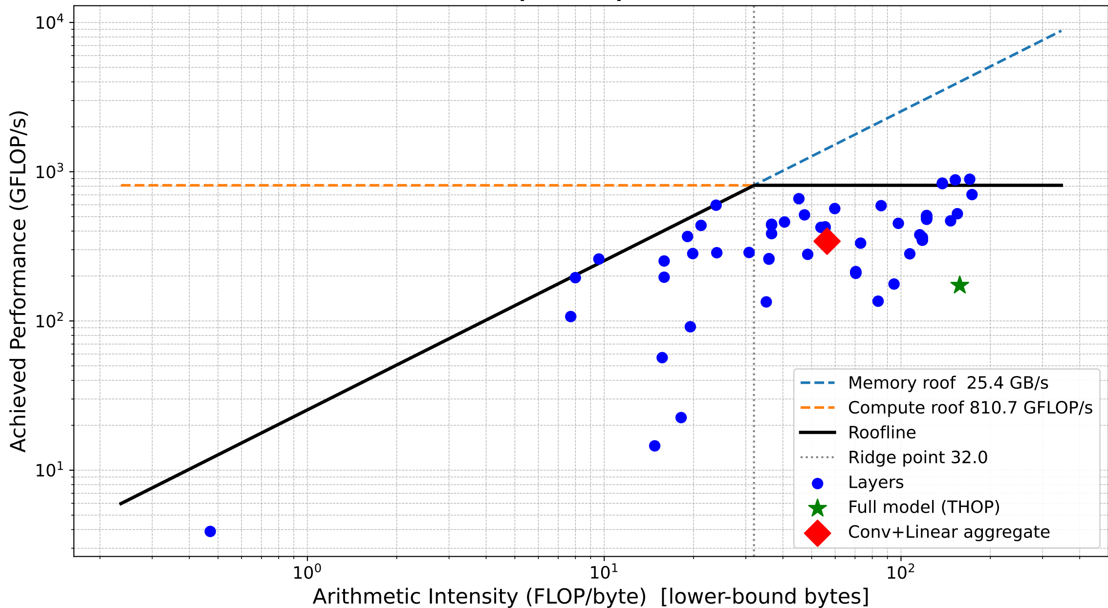
Roofline (cuda:0) — YOLOv8n
