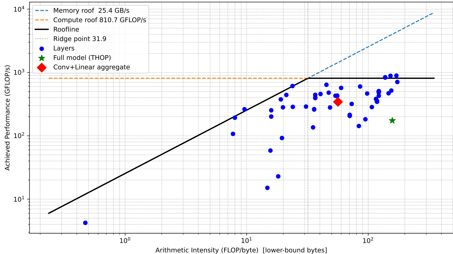
Roofline (cuda:0) — YOLOv8n
