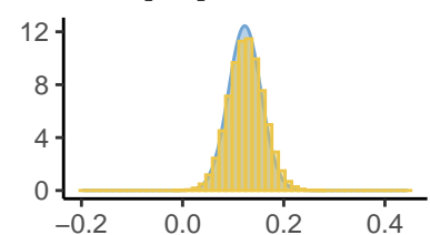
Beta[15]
