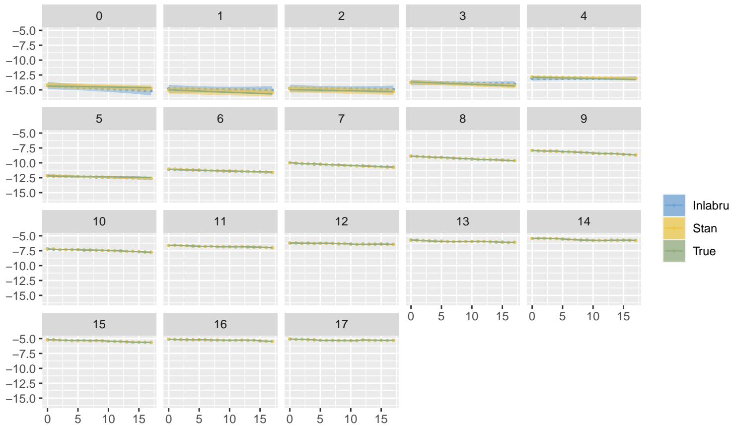
Eta – inlabru, for each age
