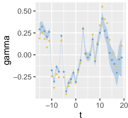
Gamma – inlabru
