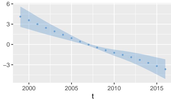
Kappa
