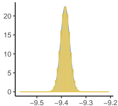
Predictor[192]
