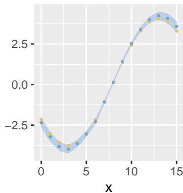
Gamma – inlabru
