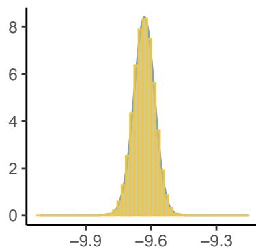
Predictor[128], Inlabru :
