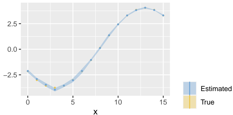
Alpha – inlabru
