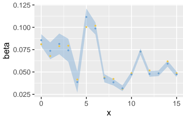
Beta – inlabru
