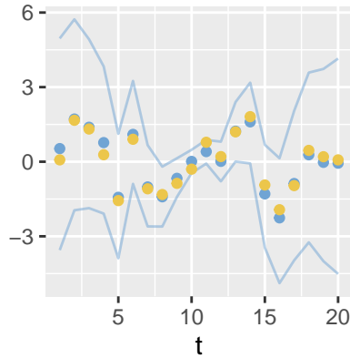
Stan – kappa
