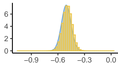
Kappa[5]
