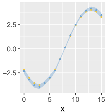
Gamma – inlabru
