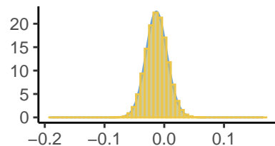
Kappa[17], Inlabru and stan
