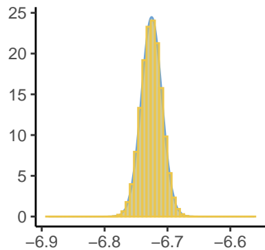
Predictor[1]
