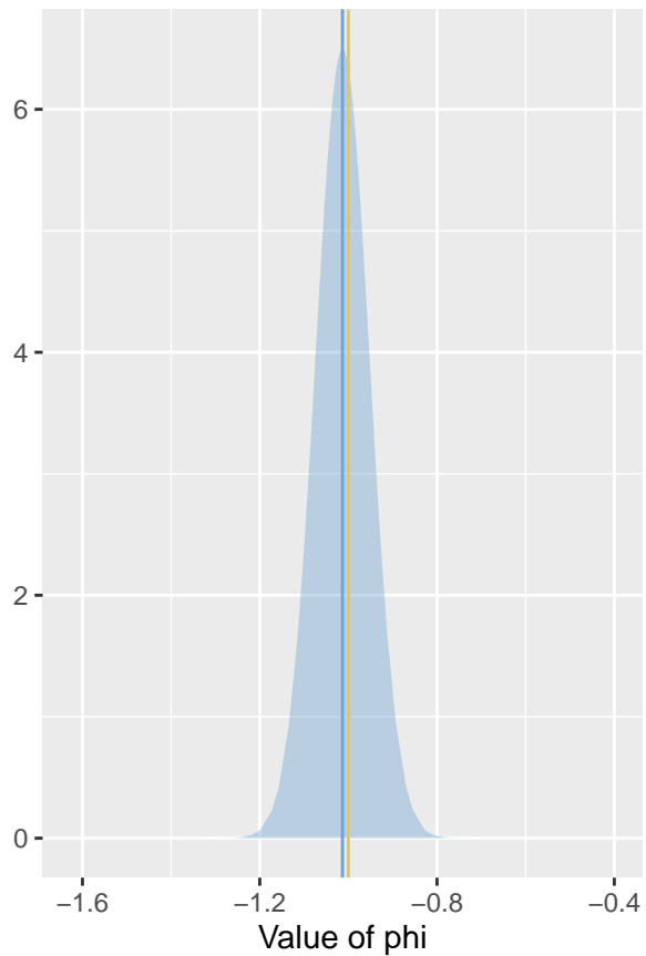
Phi – inlabru
