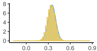
Kappa[13]
