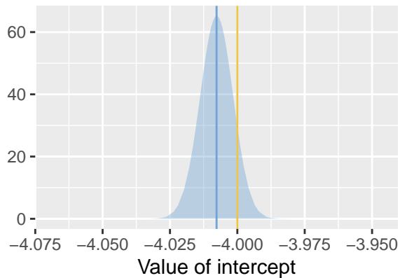
Beta – inlabru
