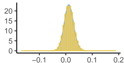
Kappa[5], Inlabru and stan
