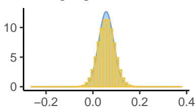
Beta[17]
