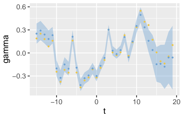
Gamma – inlabru
