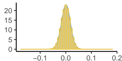
Kappa[11], Inlabru and stan
