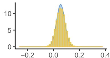
Beta[11]
