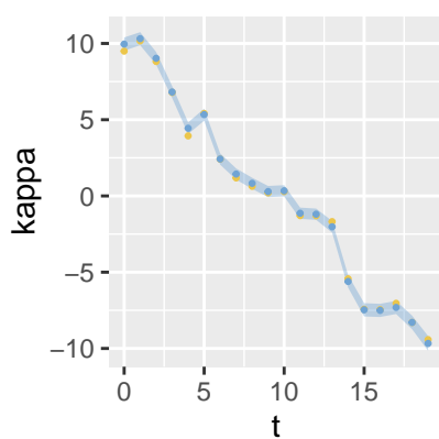
Kappa – inlabru
