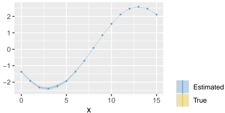
Kappa – inlabru
