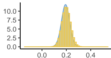
Beta[9]
