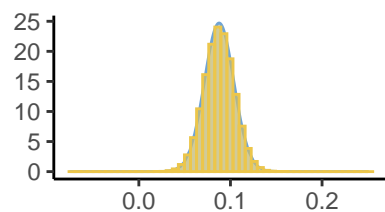
Beta[6]
