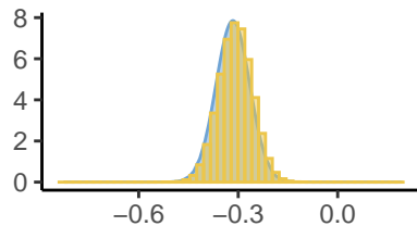
Kappa[7]
