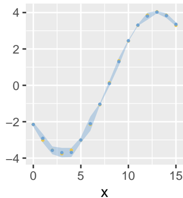
Gamma – inlabru
