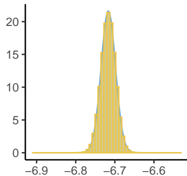
Predictor[1]
