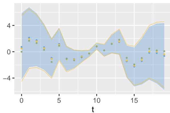
Kappa
