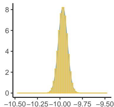
Predictor[162], Inlabru a
