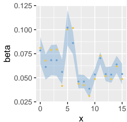
Gamma – inlabru
