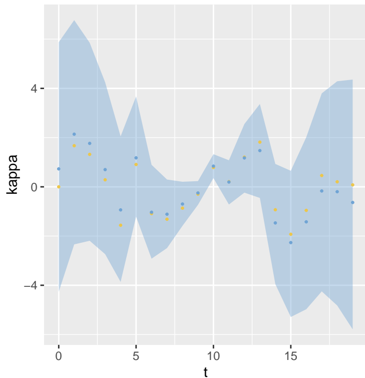
Kappa – inlabru
