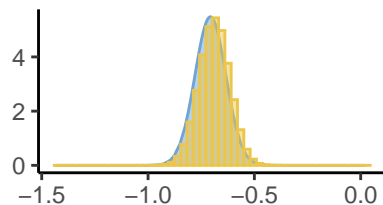
Kappa[1]
