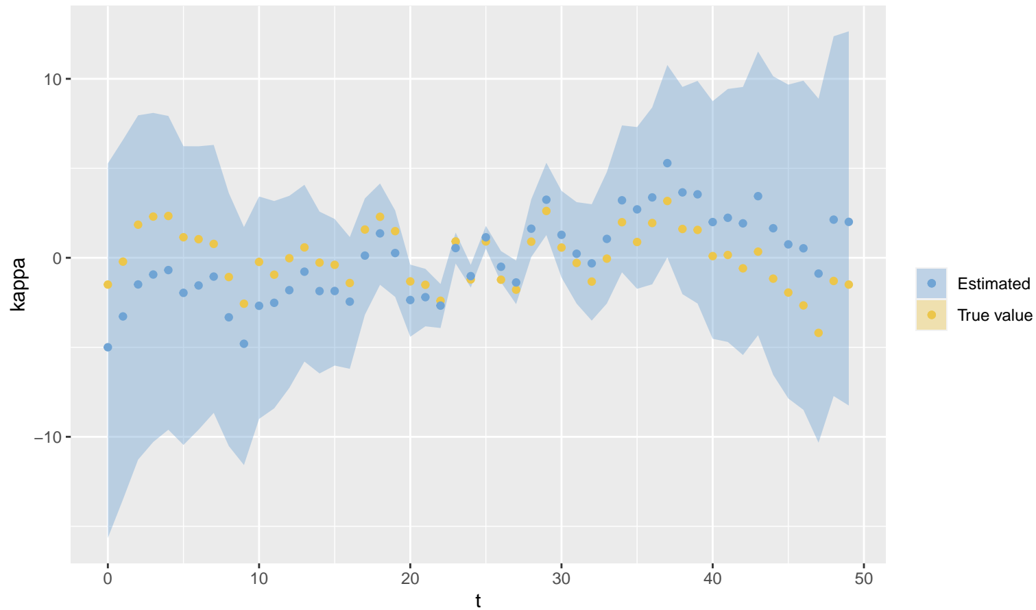
Kappa – inlabru
