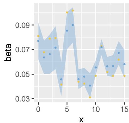
Gamma – inlabru
