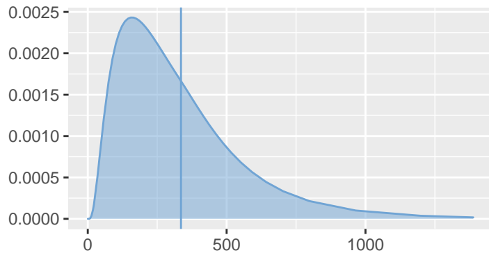
Precision of kappa
