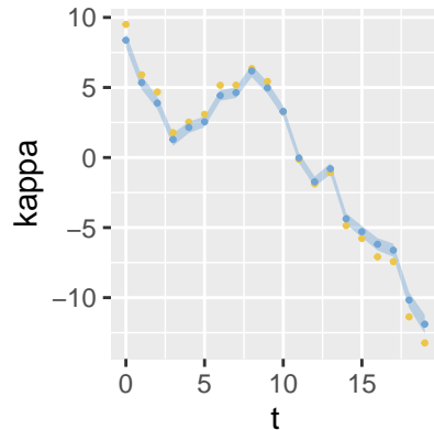
Kappa – inlabru
