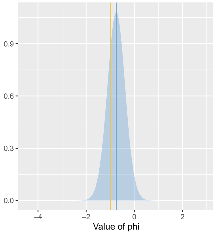
Phi – inlabru
