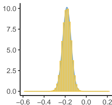
Epsilon[162], Inlabru ai
