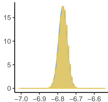
Predictor[128]
