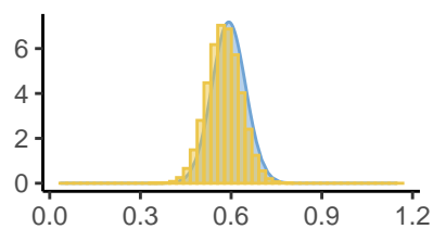
Kappa[15]
