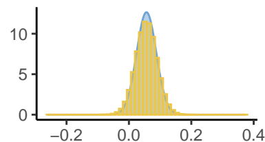
Beta[5]
