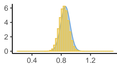
Kappa[17]
