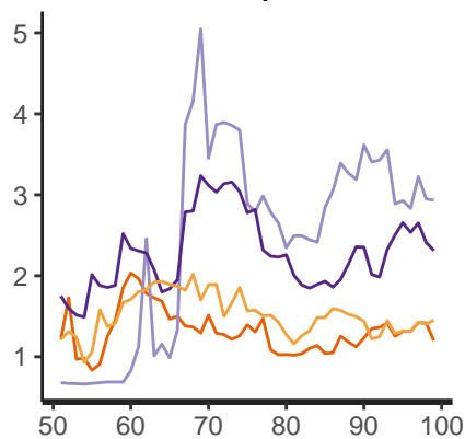
tau_epsilon
