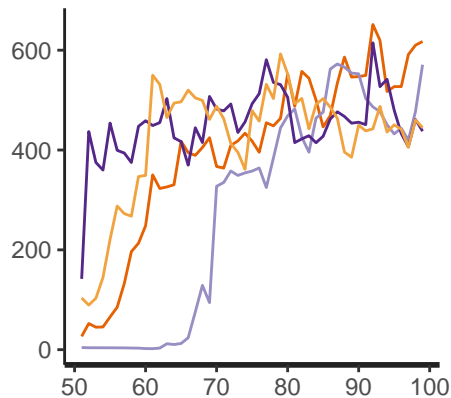
tau_epsilon
