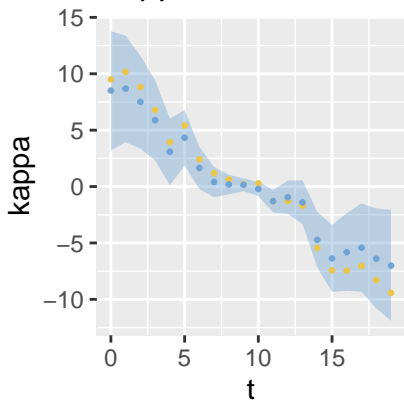
Kappa – inlabru
