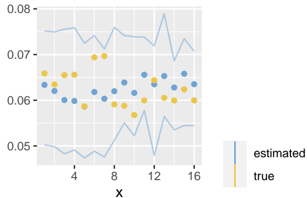
Stan – gamma
