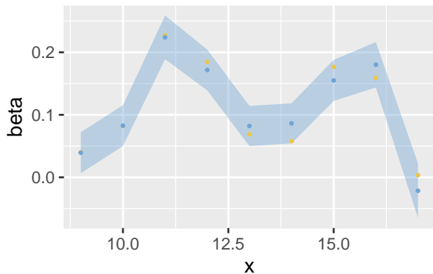
Beta – inlabru
