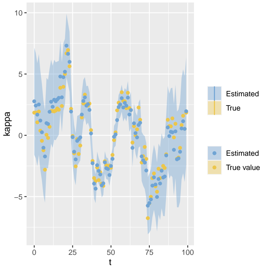
Kappa – inlabru
