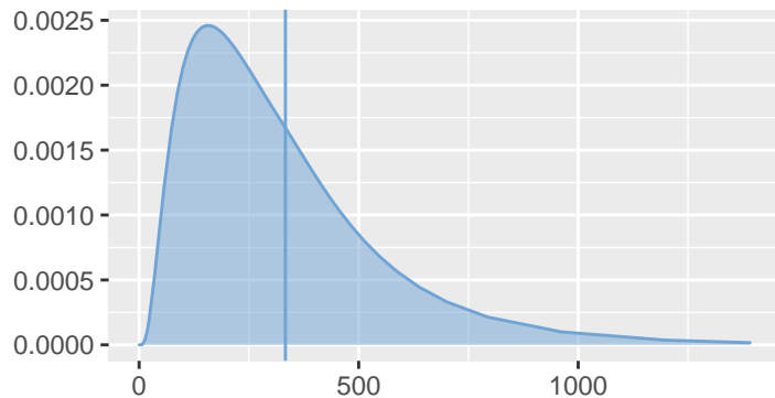
Precision of kappa
