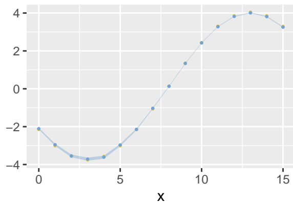
Kappa – inlabru
