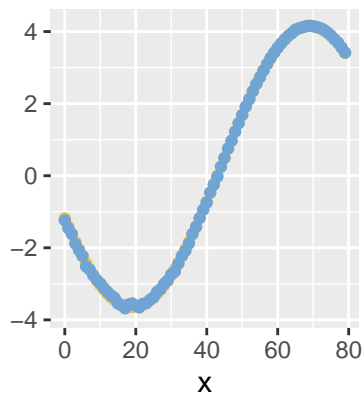
Gamma – inlabru
