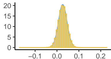
Kappa[1], Inlabru and stan
