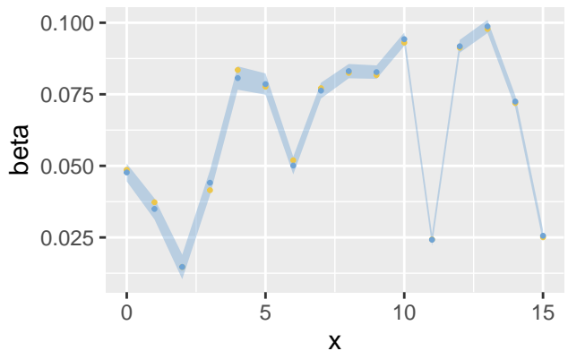
Beta – inlabru
