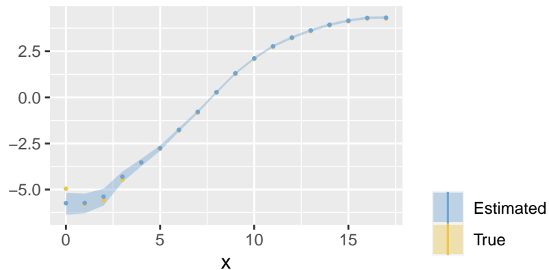
Kappa – inlabru
