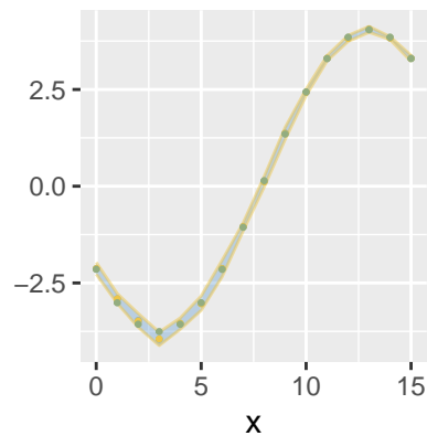
Kappa
