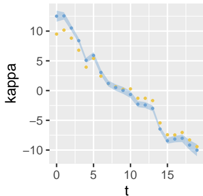
Kappa – inlabru
