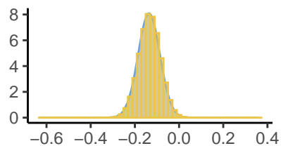
Kappa[9]
