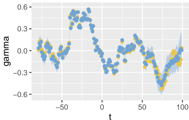
Gamma – inlabru
