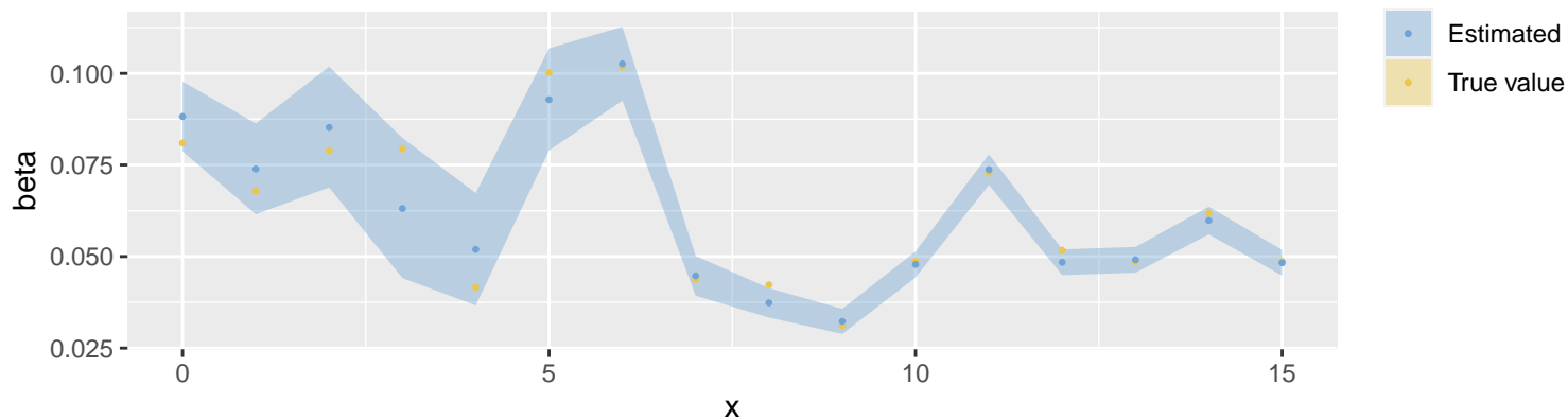
Beta – inlabru
