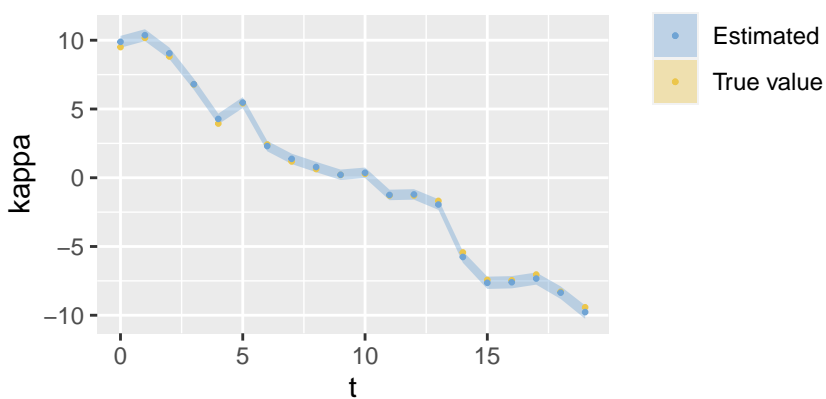
Kappa – inlabru
