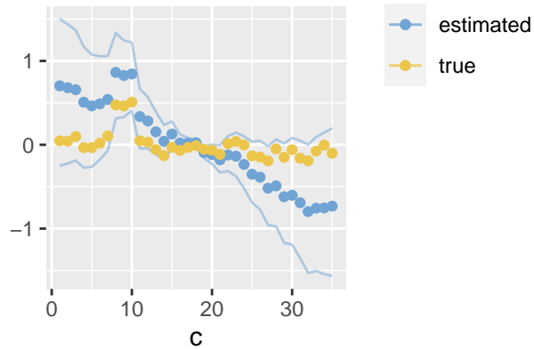
Stan – gamma
