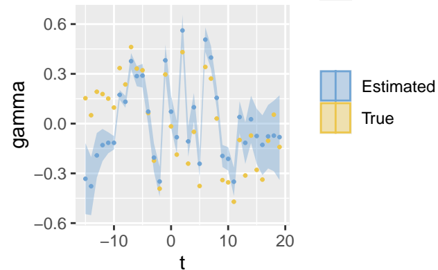
Gamma – inlabru
