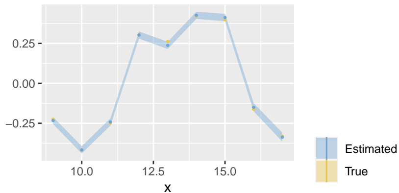
Kappa – inlabru
