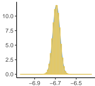
Predictor[128]
