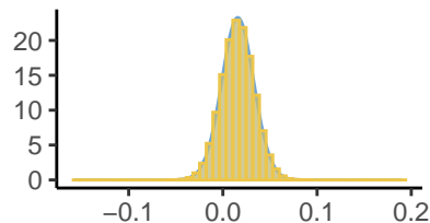
Kappa[9], Inlabru and stan
