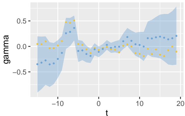
Gamma – inlabru
