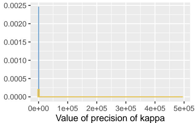
Precision of Kappa
