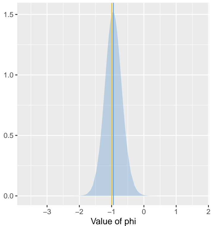
Phi – inlabru
