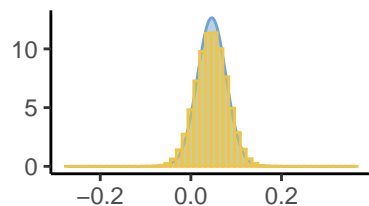
Beta[1]
