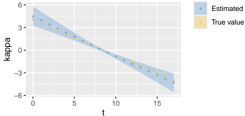
Kappa – inlabru
