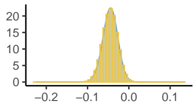
Kappa[15], Inlabru and stan
