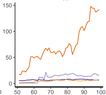
tau_kappa
