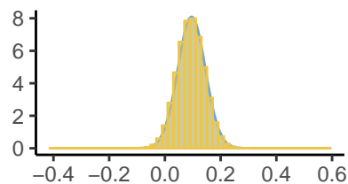
Kappa[11]
