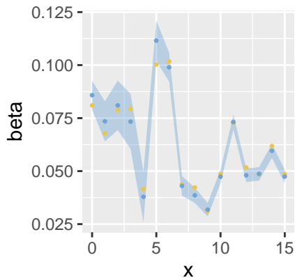
Beta – inlabru
