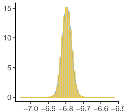
Predictor[1]
