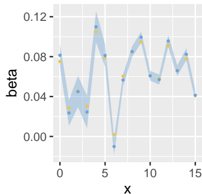
Beta – inlabru
