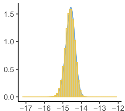
Predictor[1], Inlabru an
