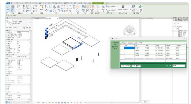
Beam: 보 4개, 체적 합계 3.428 (선택한 요소의 Revit 속성과 일치)
