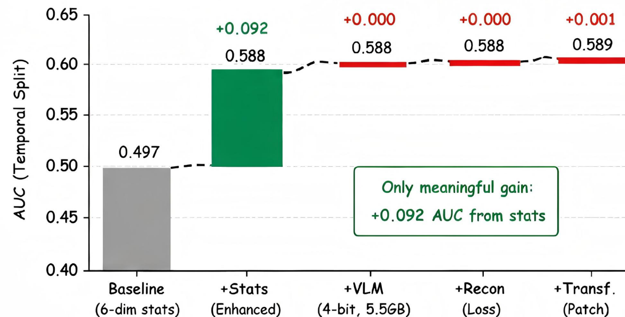
(d) Component Ablation on SWaT
