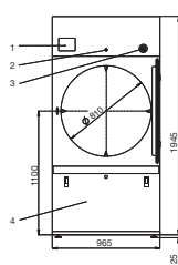
ARRIÈRE T 24 35 (VERSION VAPEUR)
