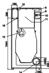
ARRIÈRE T 24 35 (VERSION VAPEUR)
