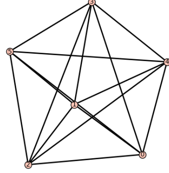
(b) K_6 .
