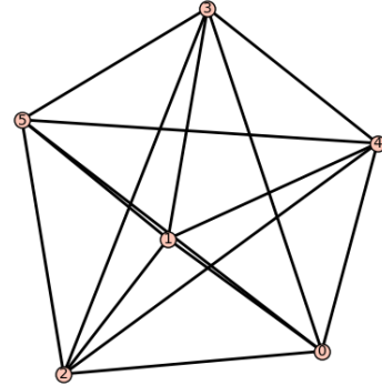
(b) K_6 .
