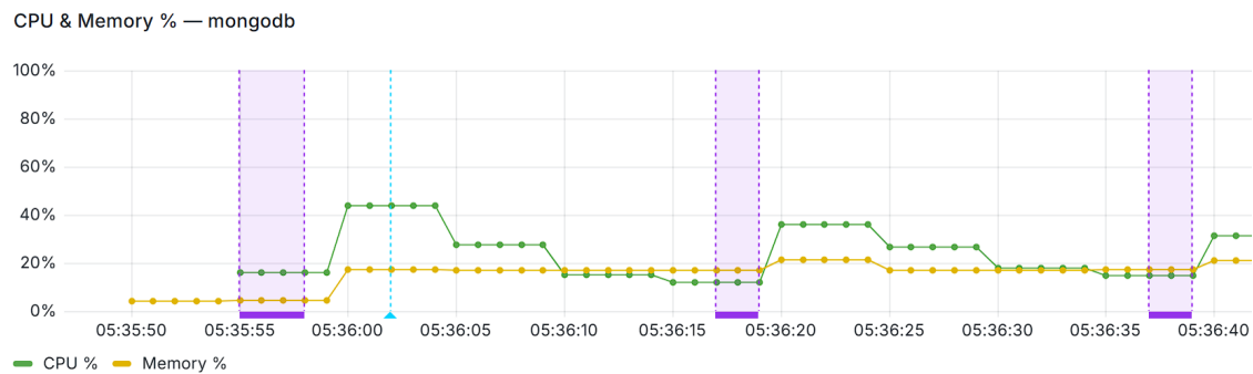
Obrázek 4.2.: Měření CPU a RAM pro test aggregate u MongoDB (zdroj: Vlastní zpracování)
