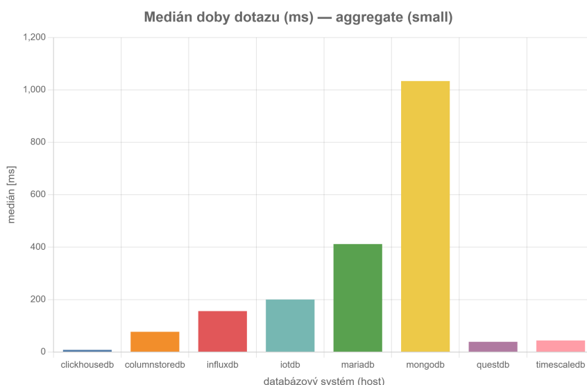
Obrázek 4.1.: Medián doby trvání dotazu aggregate na profilu small (zdroj: Vlastní zpracování)
