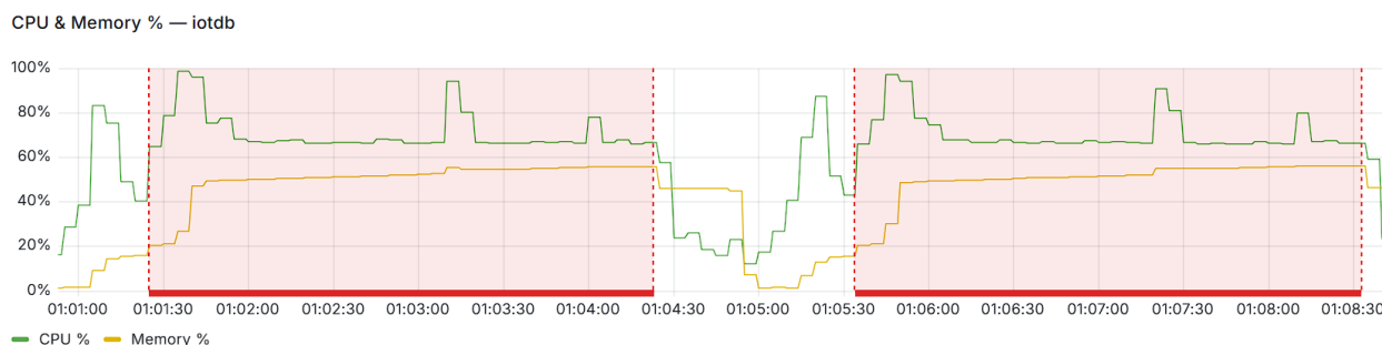
Obrázek 4.4.: Vytížení CPU a paměti Apache IoTDB během testu insert na profilu medium (zdroj: Vlastní zpracování)
