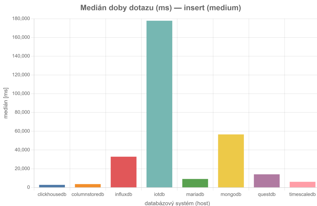
Obrázek 4.3.: Medián doby trvání dotazu insert na profilu medium (zdroj: Vlastní zpracování)
