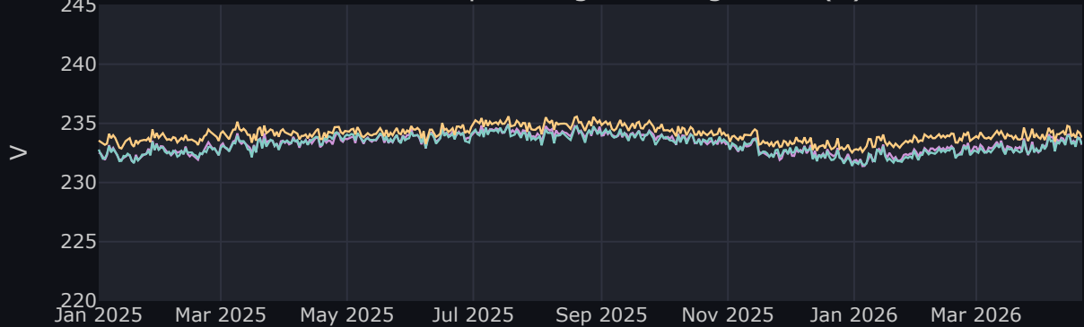
④ Phasenspannungen — Allgemein (V)
