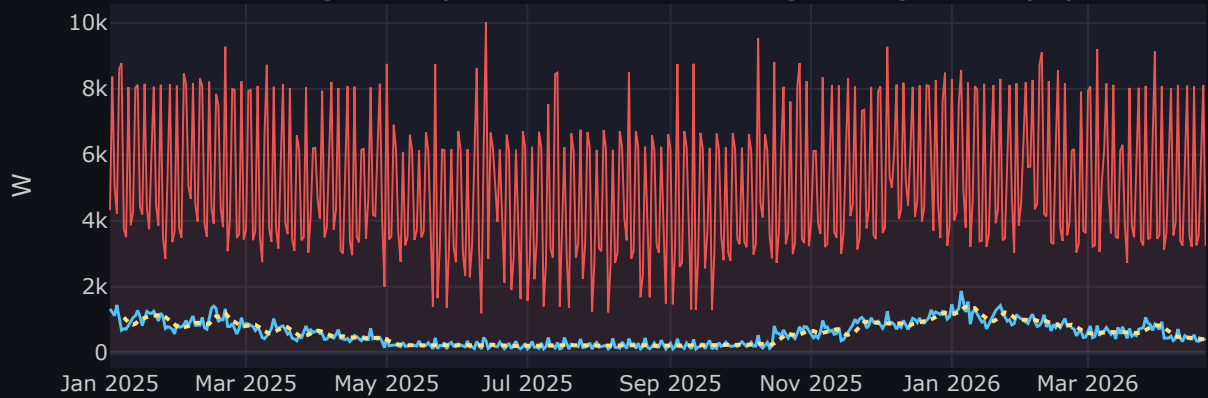
③ Tägliche Spitzen- und Ø-Leistung — Allgemein (W)
