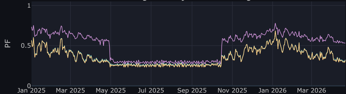
⑤ Leistungsfaktor je Phase — Allgemein
