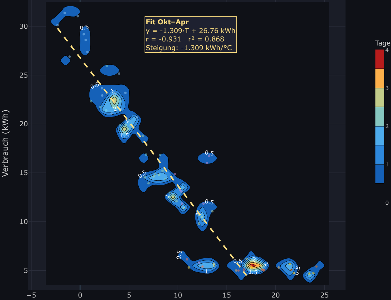
③ 4-Wochen Glättung: Verbrauch & Temperatur
