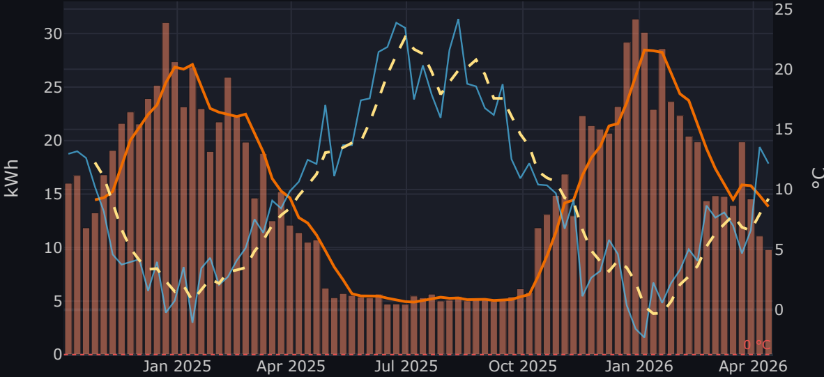
① Wochenmittel: Temperatur (°C) vs. Verbrauch Allgemein (kWh)
