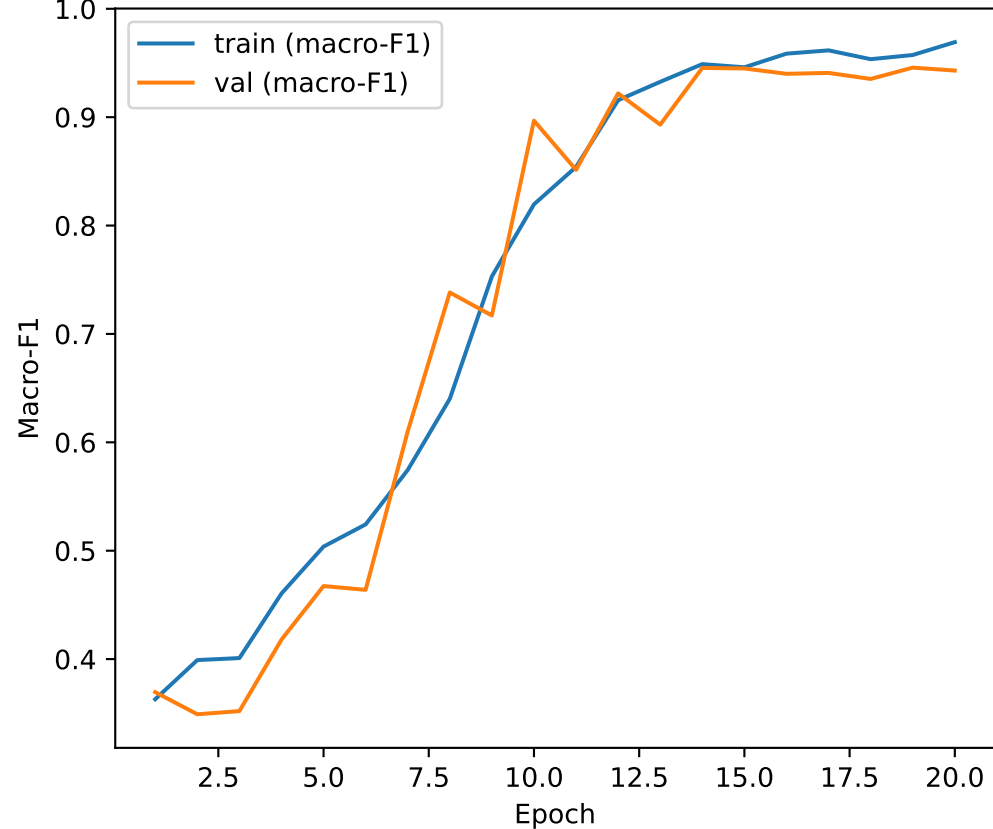
Macro-F1 per Epoch
