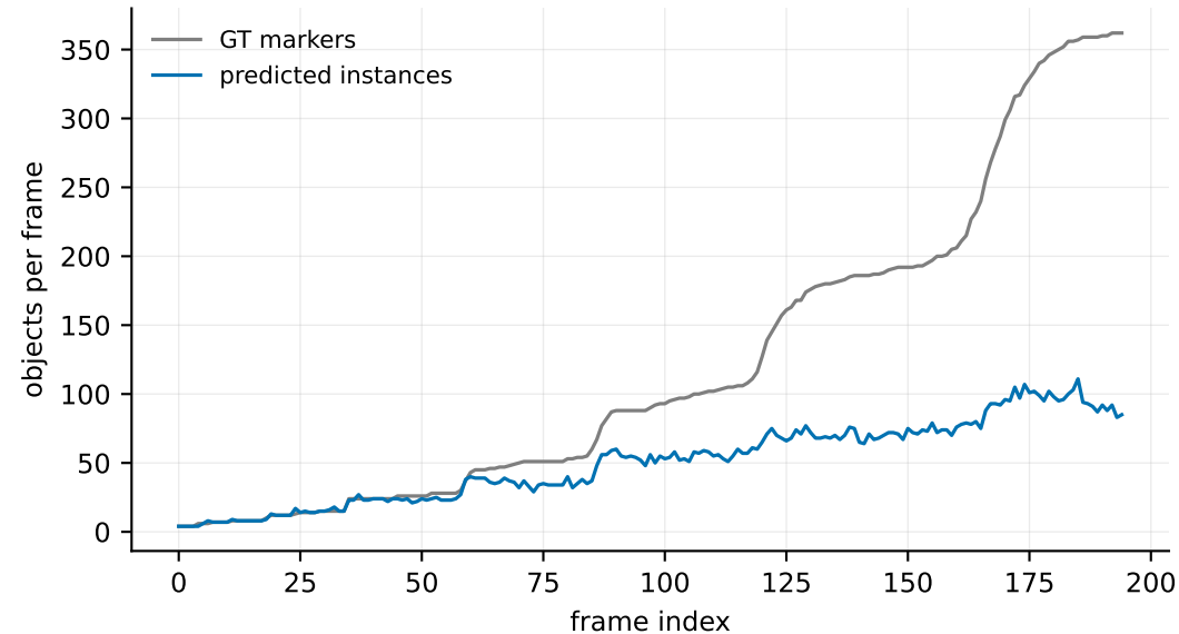
Detections vs GT markers (nnU-Net, seq01)
