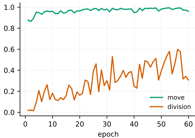
validation F1
