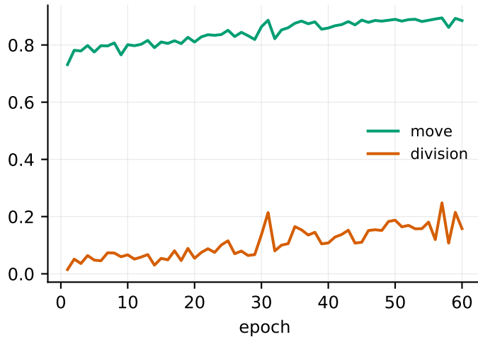
validation F1
