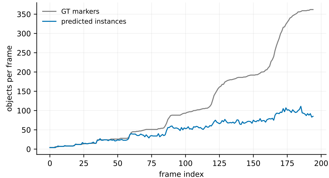
Detections vs GT markers (nnU-Net, seq01)
