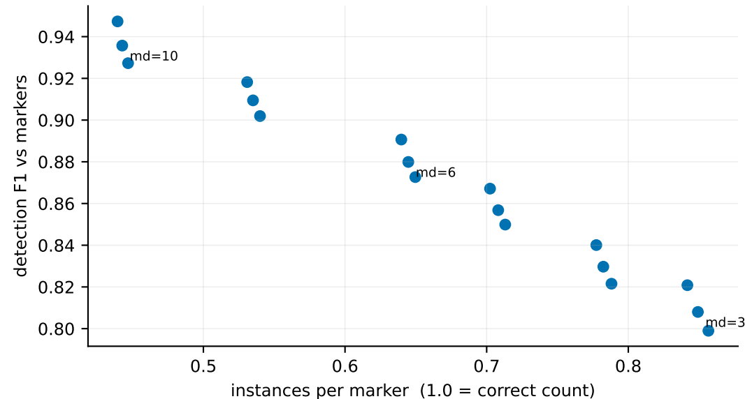
F1 rewards under-segmentation
