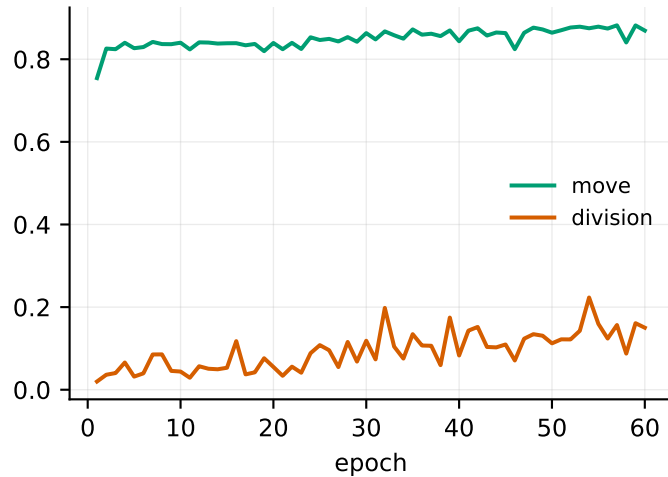
validation F1
