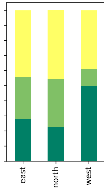
loo_0.6
