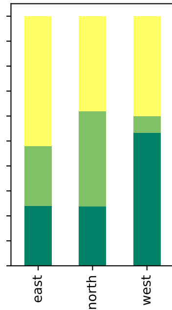
loo_0.6
