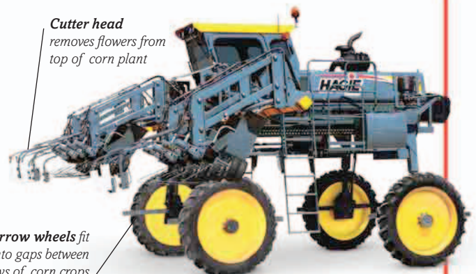
Hagie 204SP Detassler USA 2013
