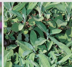
S. officinalis
