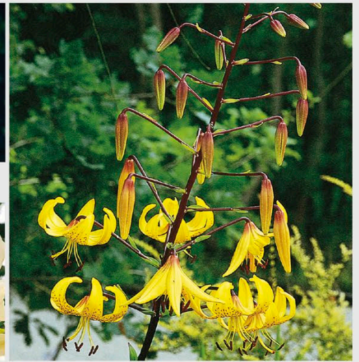
L. leichtlinii
