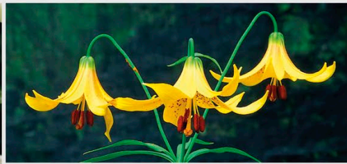
L. canadense
