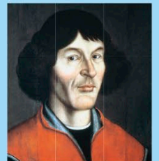
Nicolaus Copernicus
