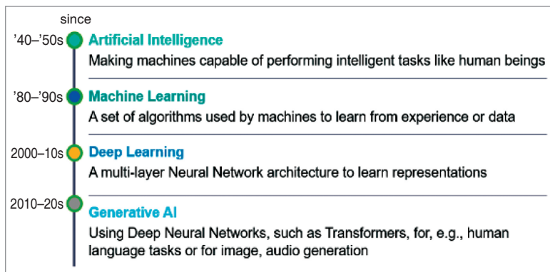
Fig. 1: Generative AI
