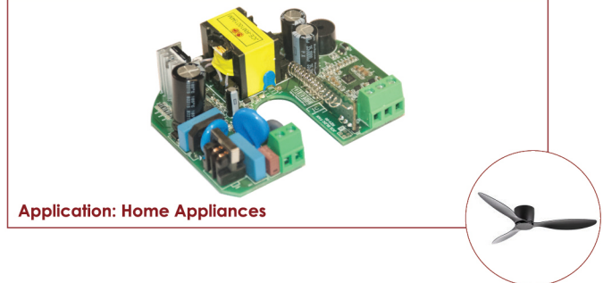
BLDC CEILING FAN CONTROLLER
