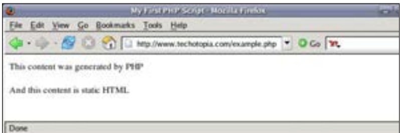
PHP Output
