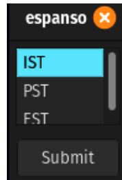
Figure 3: Espanso list
