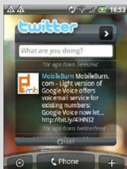
▲ Twitter app
