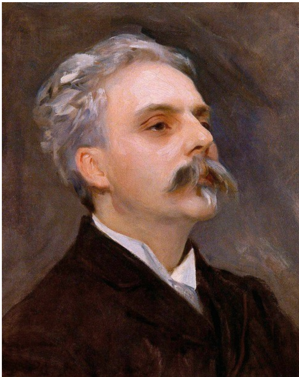
GABRIEL FAURE
