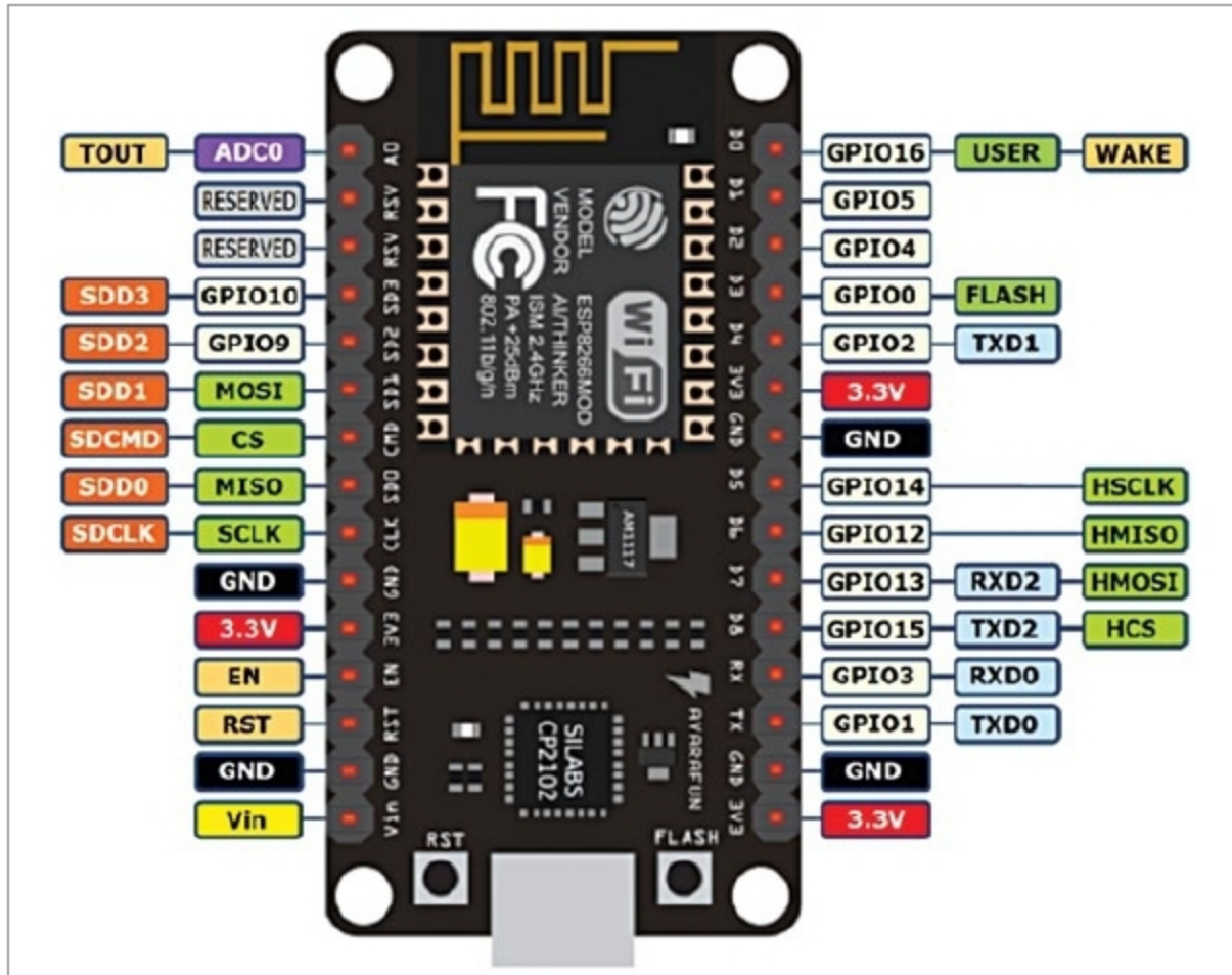
Fig. 4: NodeMCU module pin details
