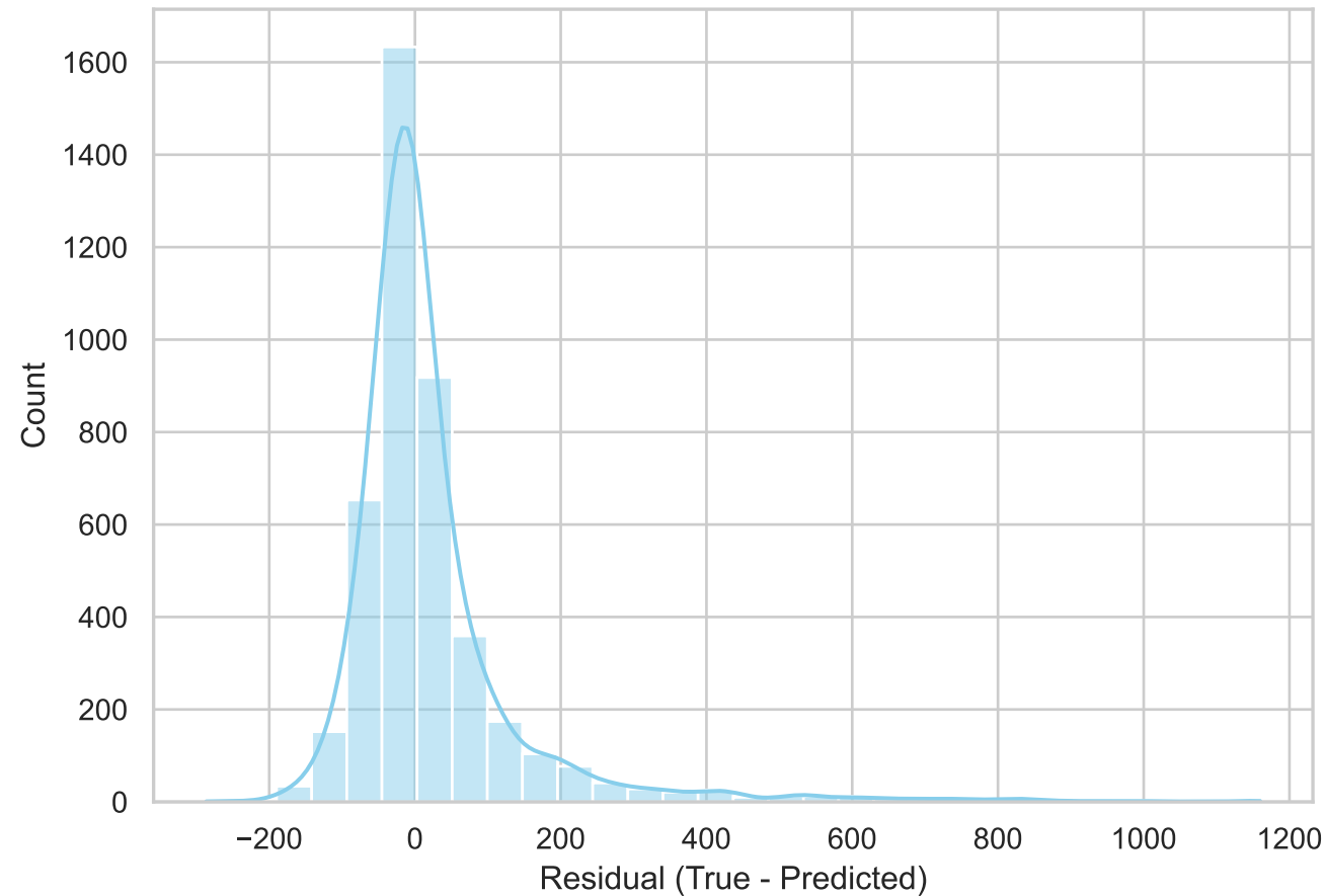
Big Tier: Residuals Distribution
