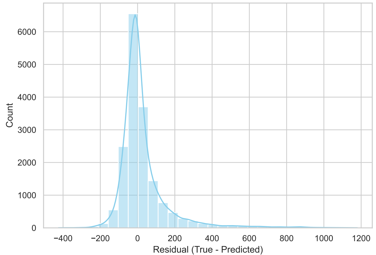
Medium Tier: Residuals Distribution
