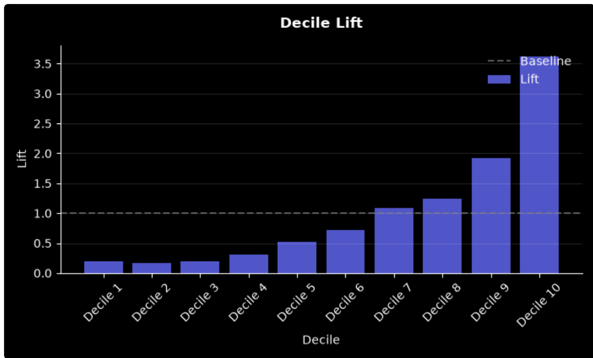
CHART_DECILE_LIFT
