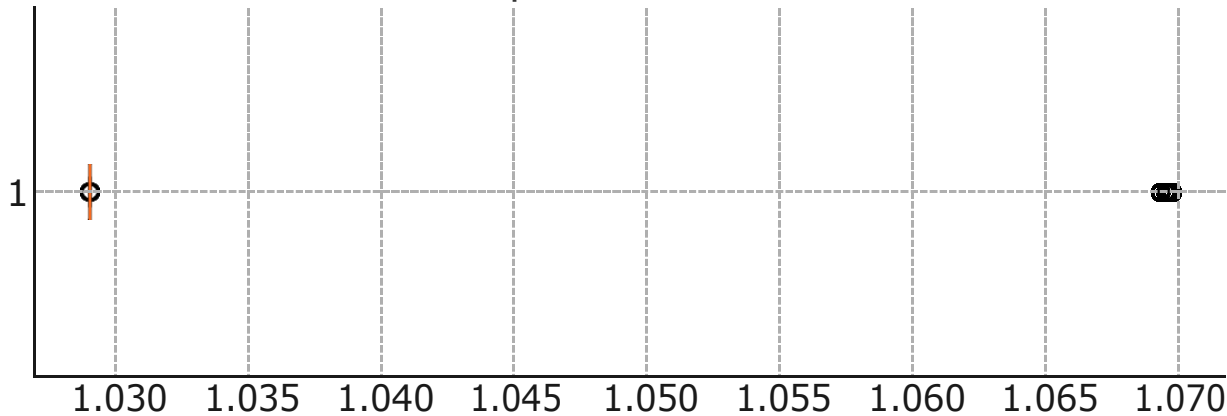
Boxplot: Item Code
