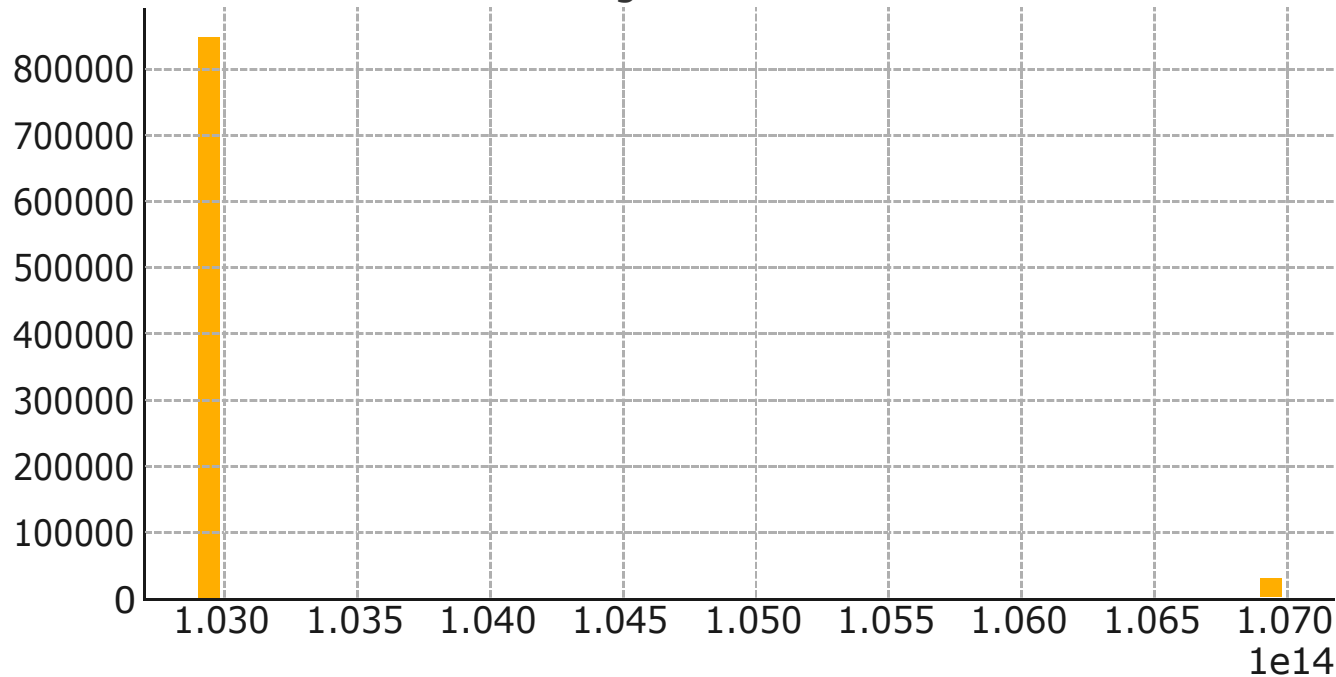
Histogram: Item Code
