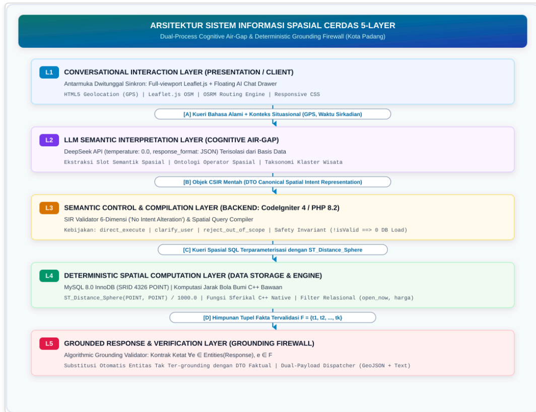
Gambar 1. Evolusi Arsitektural: Transformasi dari Three-Tier Web GIS Konvensional (DTE Explorer, Afnarius dkk., 2026) Menuju Sistem Informasi Spasial 5-Layer dengan Sandboxed Cognitive Interpretation dan Algorithmic Grounding Validator.
