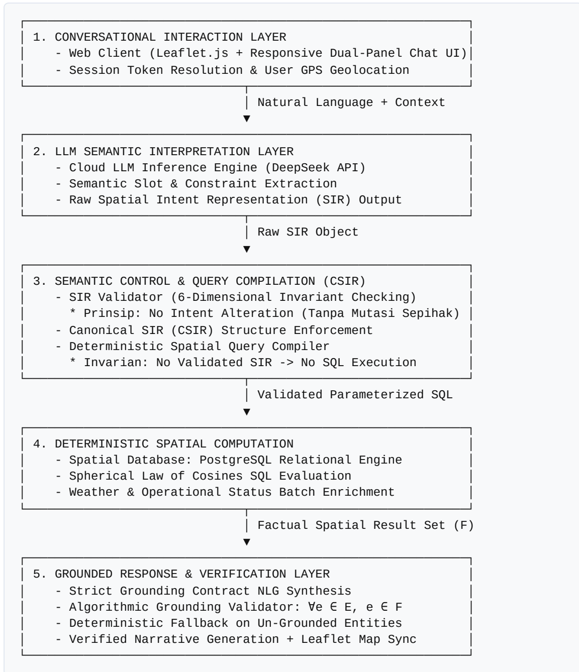
Gambar 1. Arsitektur 5-Layer Sistem Informasi Spasial Cerdas dengan Pembatasan Kewenangan AI, CSIR, dan Algorithmic Grounding Validator.
