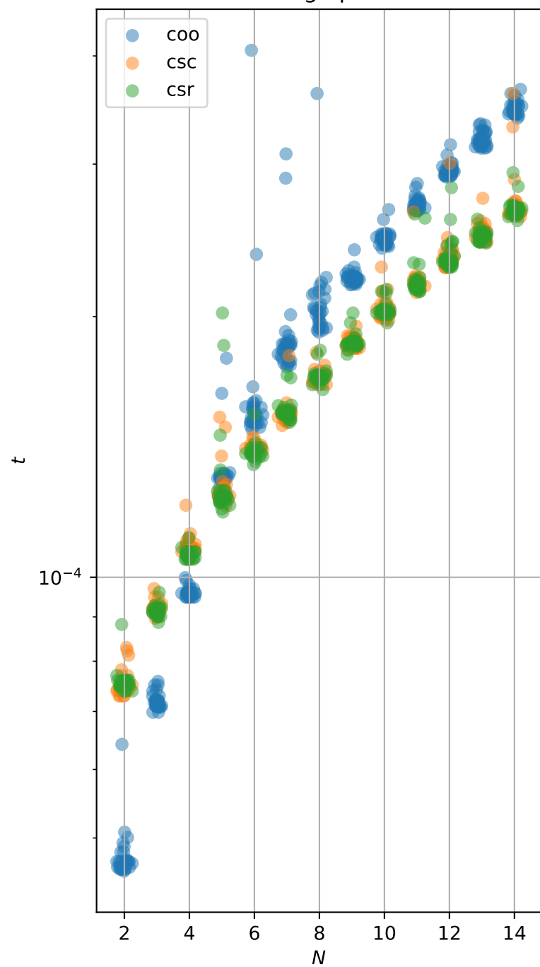
Gathering op chains
