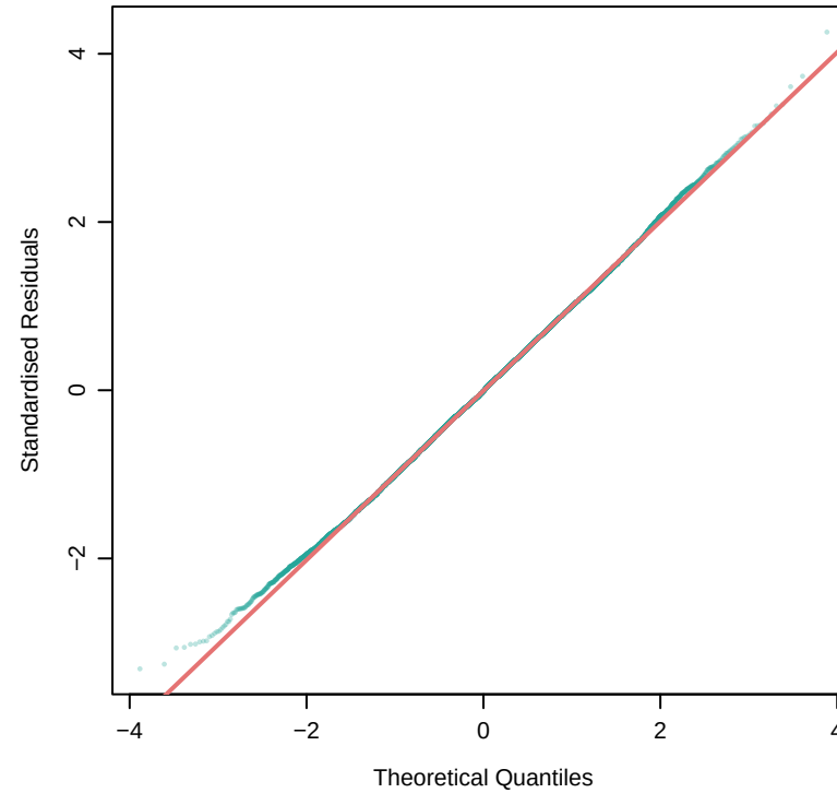
Normal Q-Q
