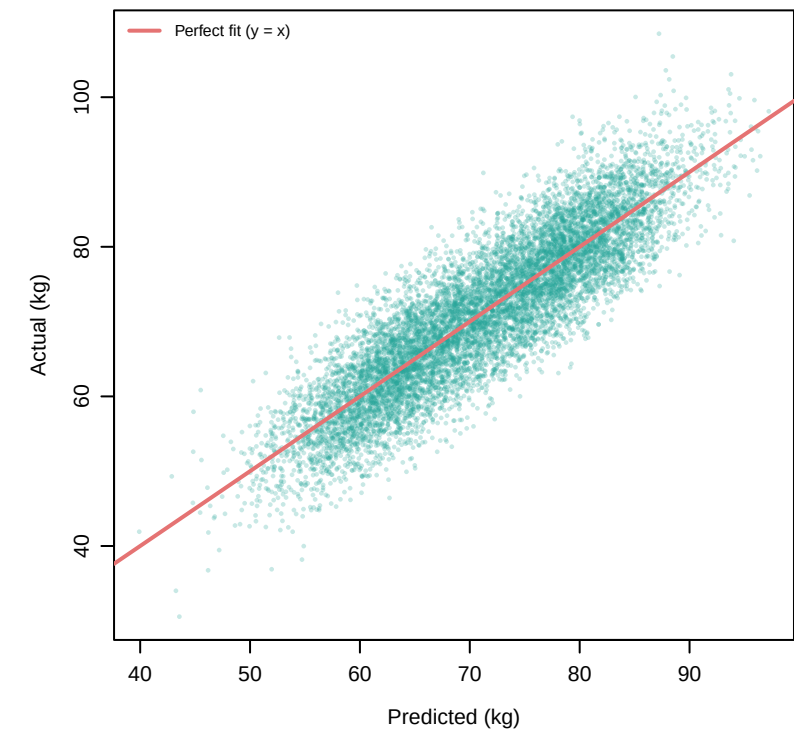
Actual vs Predicted Weight
