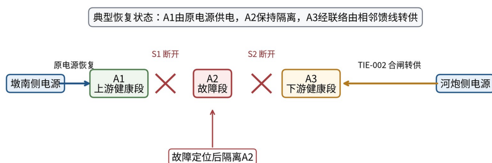
图 6-1 TIE-002 分段隔离与联络转供示意
