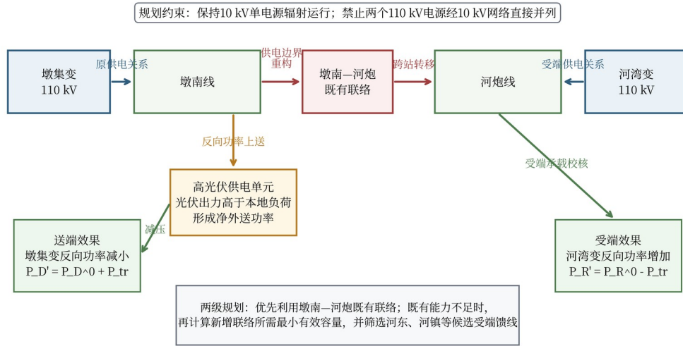
图 6-1 墩南—河炮既有联络高光伏跨站供电边界重构示意
