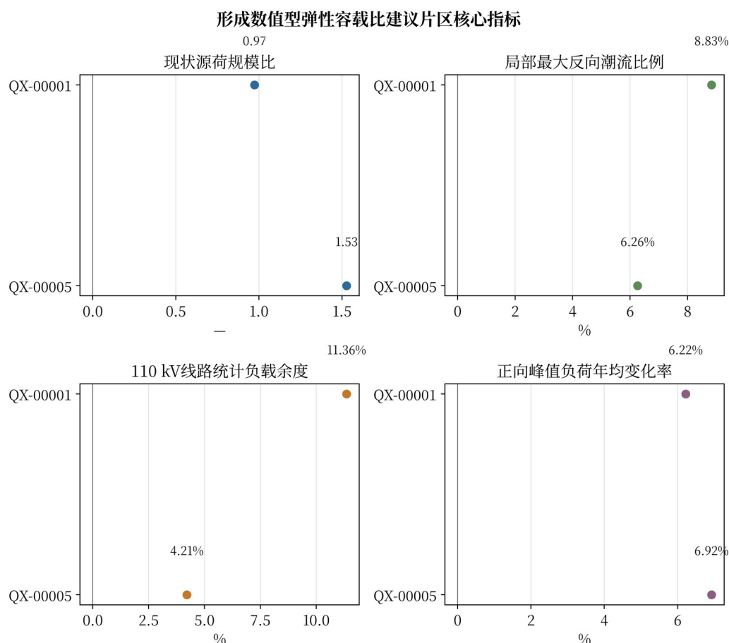
图 3-1 形成数值型弹性容载比规划控制值建议片区四项核心运行指标
