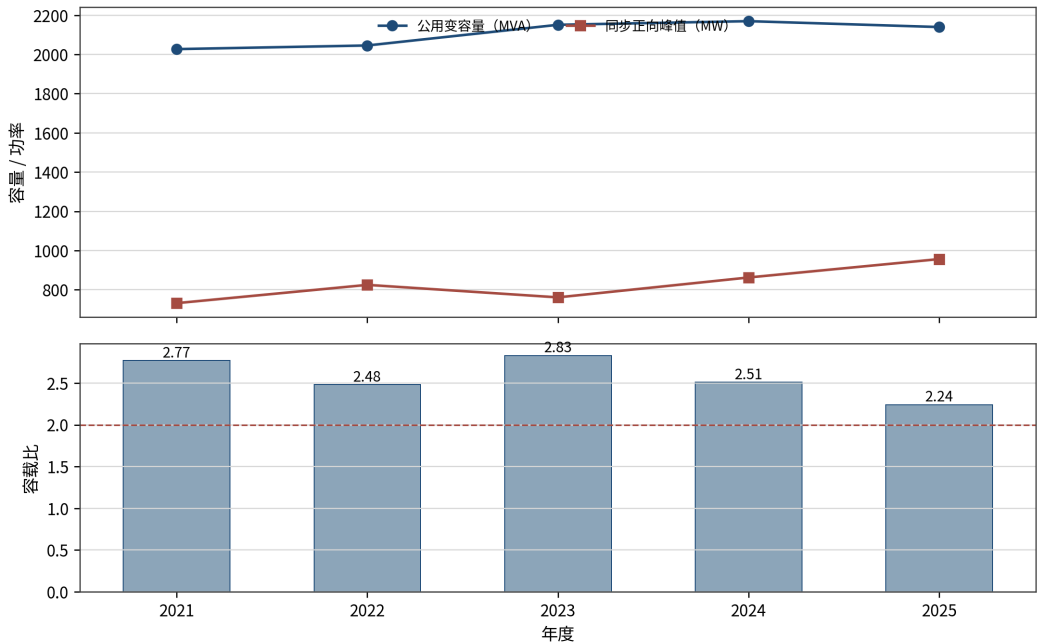
图 3-2 QX-00005 片区 110 kV 容量、同步峰值与容载比变化
