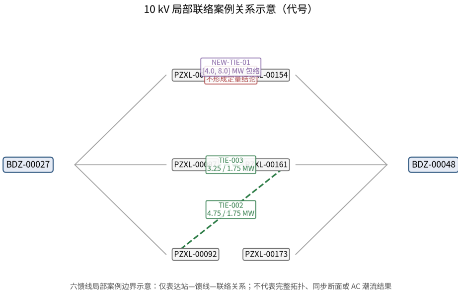
图 6-2 10 kV 局部联络案例边界
