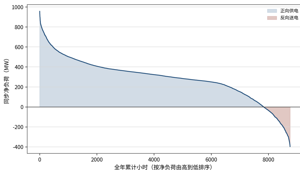
图 3-3 QX-00005 片区 2025 年 110 kV 同步净负荷持续曲线
