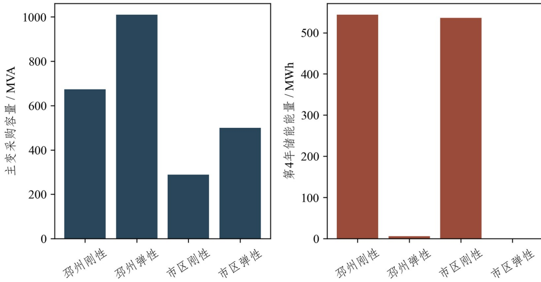
图 5-3 主变采购与储能配置对照
