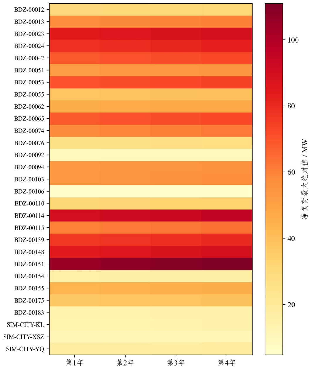
图 3-8 市区逐站仿真年度净负荷最大绝对值
