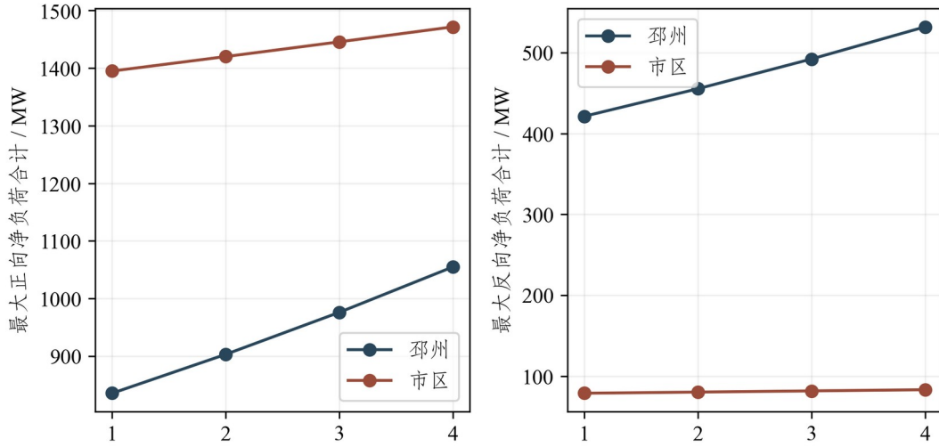
图 3-4 两地区仿真年度站级正反向净负荷
