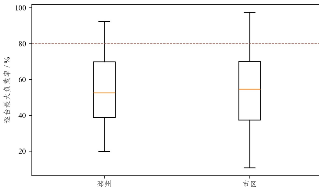
图 3-3 邳州和市区逐台主变最大负载率分布
