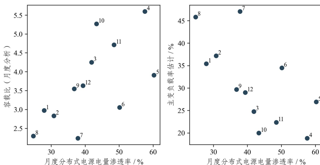
图 3-6 邳州月度分布式电源电量渗透率与容量压力关联
