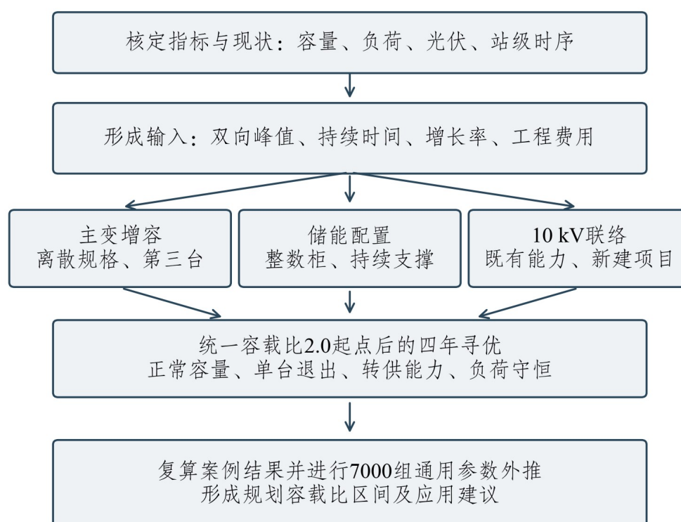
图 1-1 逐年规划计算与推荐矩阵形成过程
