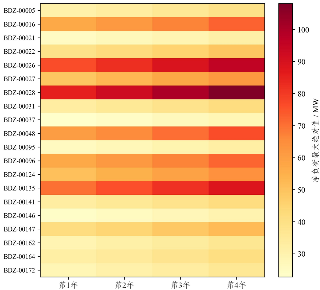
图 3-7 邳州逐站仿真年度净负荷最大绝对值
