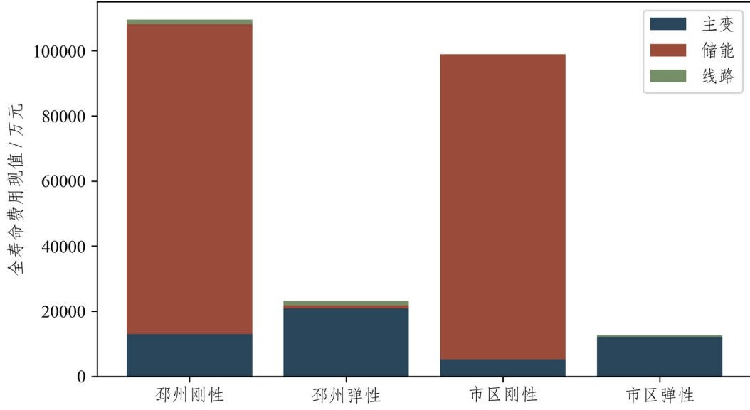
图 5-2 各规划方案全寿命费用构成
