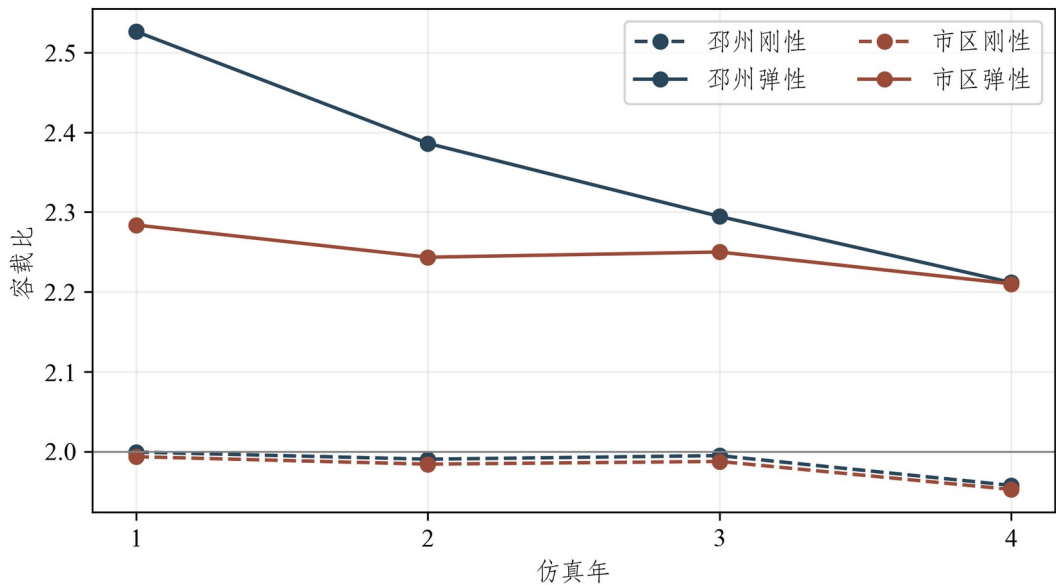
图 5-1 邳州和市区逐年容载比
