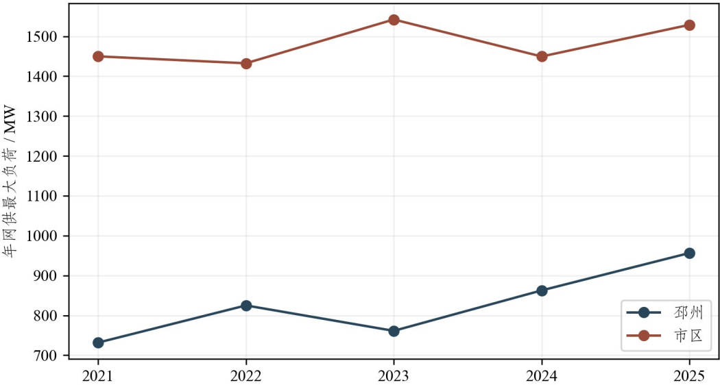
图 3-1 邳州和市区年网供最大负荷
