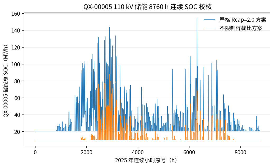
图 6-1 QX-00005 储能 8760 h 连续 SOC 校核
