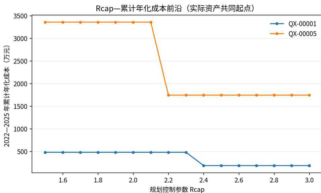
图 4-1 110 kV 片区 Rcap—累计年化成本弹性前沿
