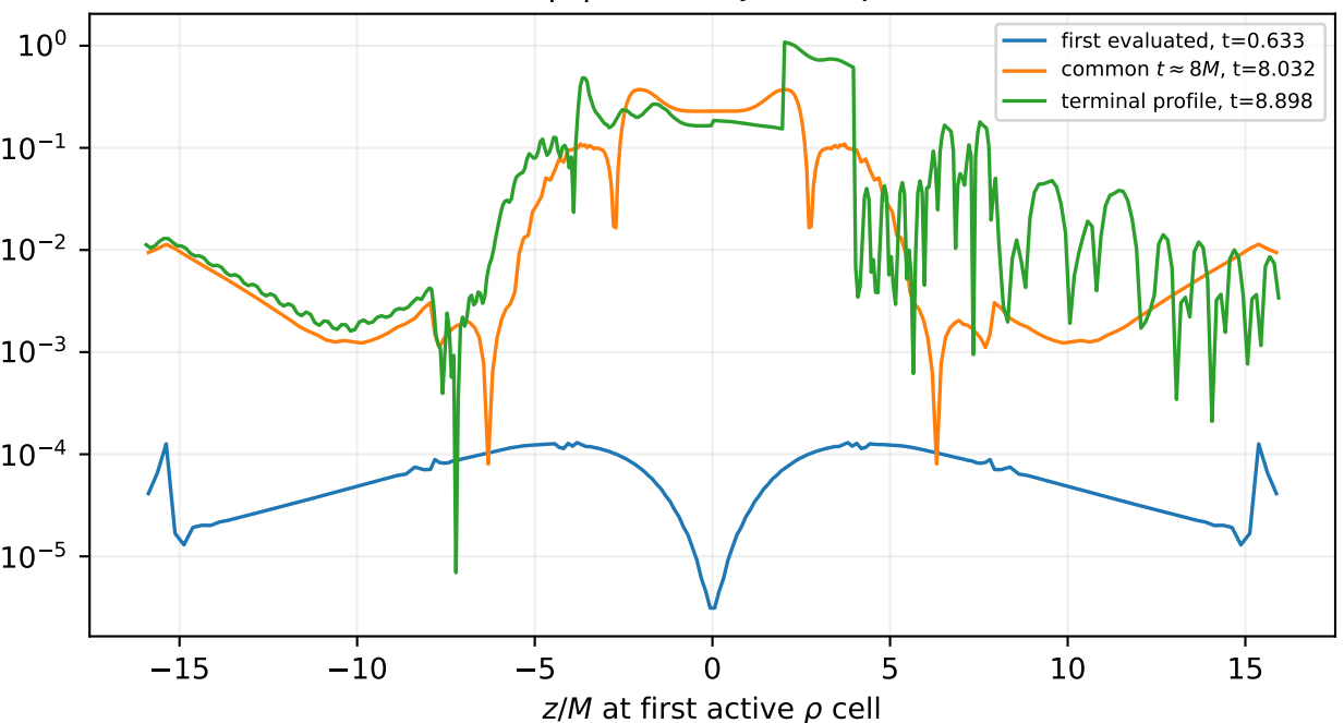
local \sqrt{K_{ij}K^{ij}} : axis-adjacent profile
