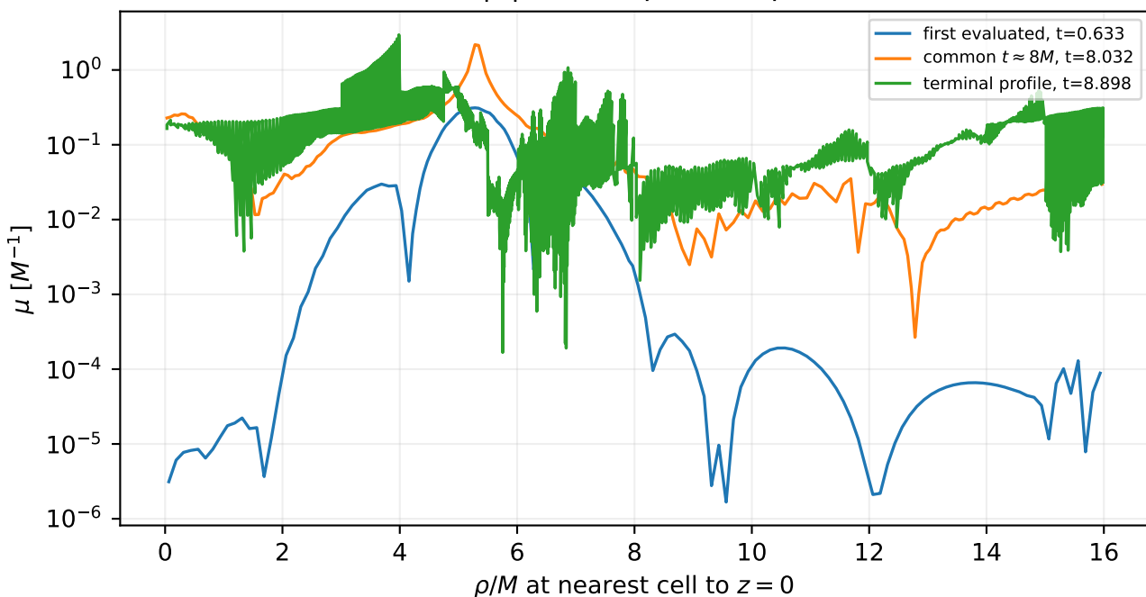
local \sqrt{K_{ij}K^{ij}} : near-equatorial profile
