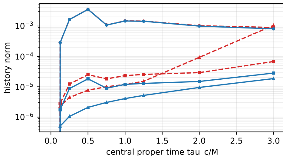
M-norm2
