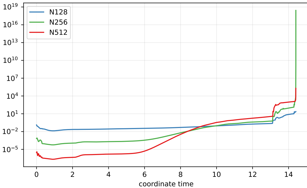
M-norm2
