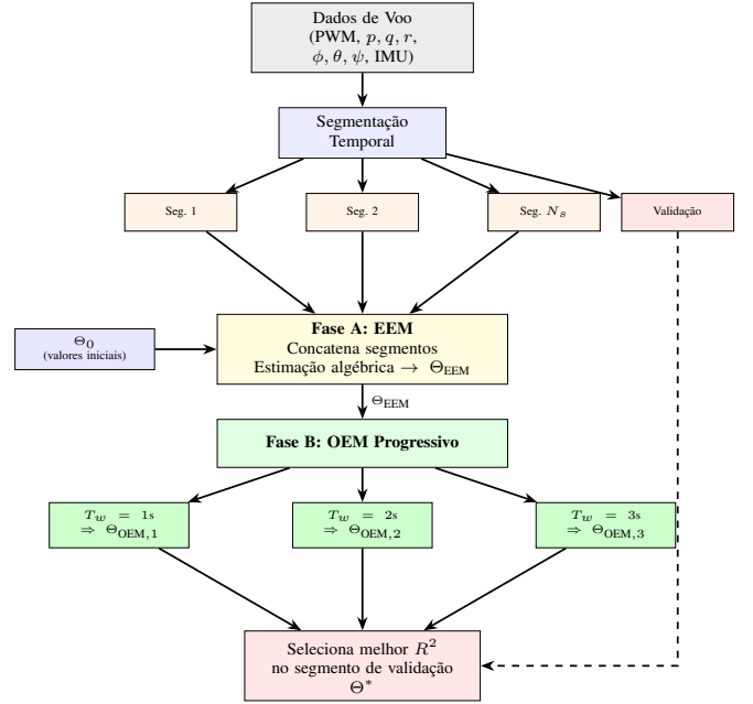
Fig. 9. Diagrama do processo de identificação por OEM com multijanelas progressivas. A partir dos valores iniciais \Theta_0 , a Fase A (EEM algébrico) fornece \Theta_{EEM} , que inicializa a Fase B (OEM com janelas de duração crescente); cada janela gera um modelo \Theta_{OEM,i} , e o melhor conjunto de parâmetros \Theta^* é selecionado com base no R^2 do segmento de validação.
