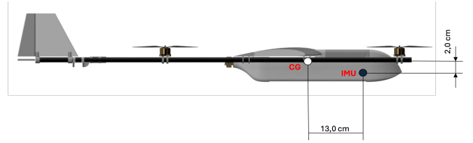
Fig. 12. Desalinhamento da IMU em relação ao CG.
