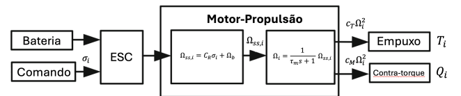
Fig. 5. Diagrama de blocos do modelo do motor: o ESC converte o comando normalizado \sigma_i em velocidade angular de regime permanente (Equação (4)), filtrada pela dinâmica de primeira ordem (Equação (5)) e transformada em empuxo e contra-torque (Equação (6)). Adaptado de [13].
