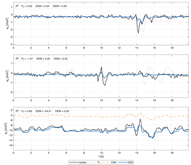
Fig. 15. Acelerações (força específica da IMU): comparação das respostas dos modelos P_0 , EEM e OEM final às medições, no segmento de validação.
