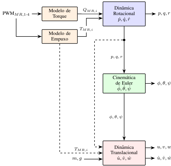
Fig. 13. Diagrama de blocos do modelo dinâmico do VANT. As entradas PWM alimentam os modelos de empuxo e torque. Linhas tracejadas indicam sinais que alimentam a dinâmica translacional.
