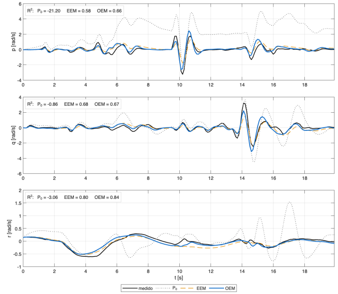
Fig. 14. Velocidades angulares: comparação das respostas dos modelos P_0 , EEM e OEM final às medições, no segmento de validação.
