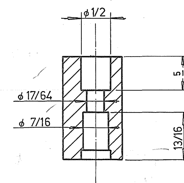
CORTE A-A
